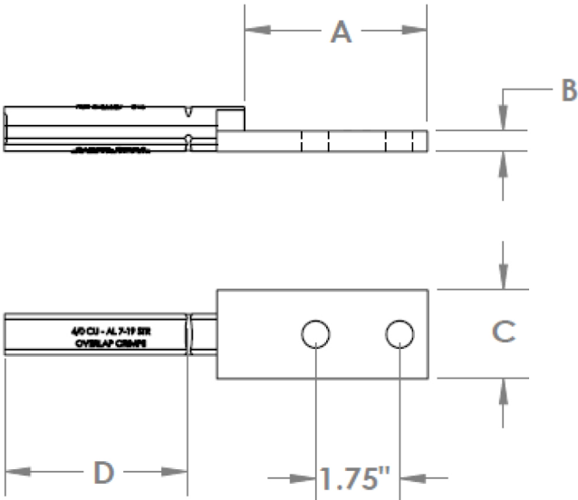
No Hardware (-NH) Option
